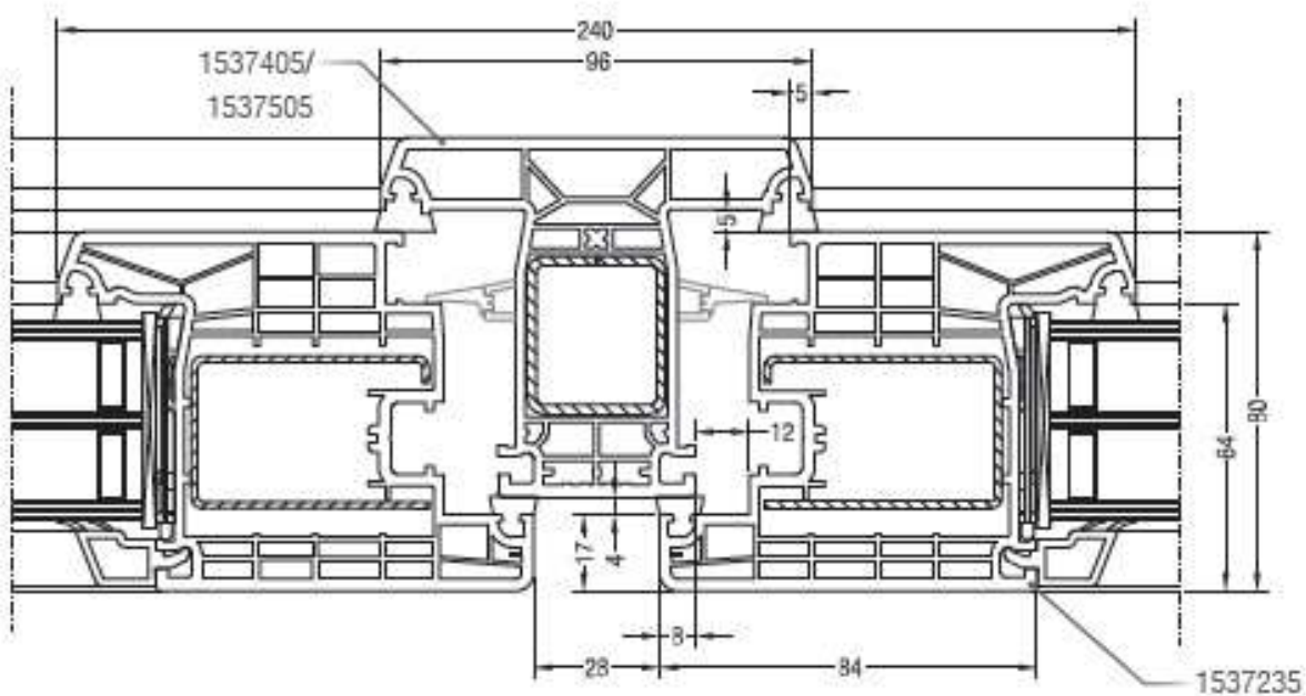
Sezione nodo- anta dritta/arrotondata - 2 ante
